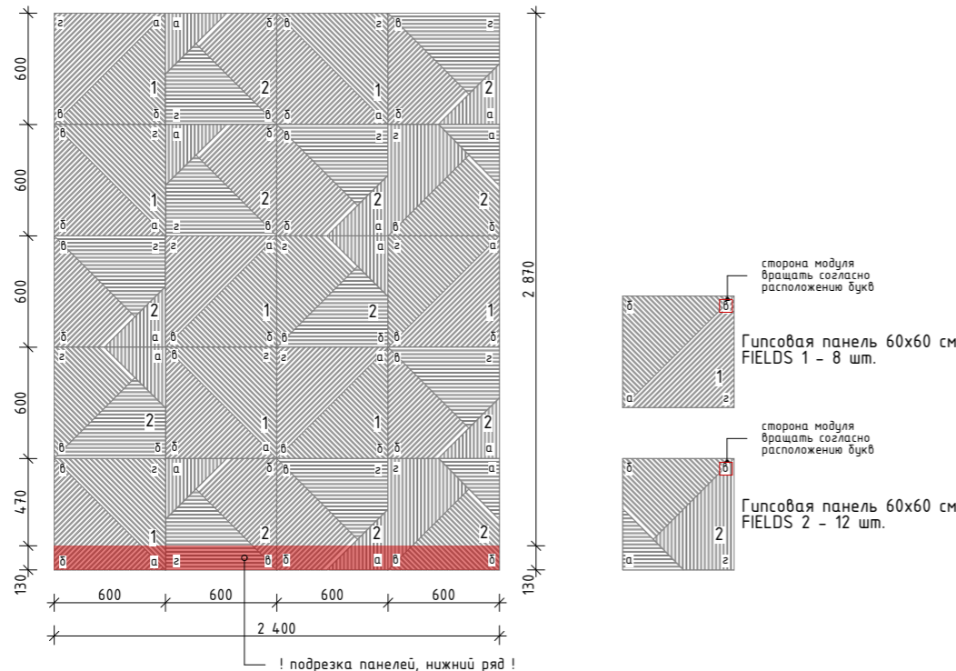
СХЕМА РАСКЛАДКИ ГИПСОВЫХ ПАНЕЛЕЙ
